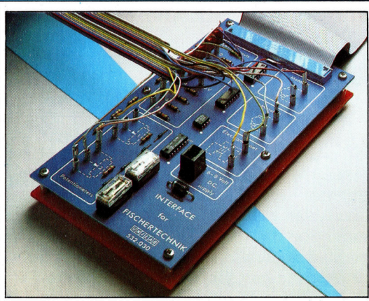
Interface Über das Unilab-Interface laufen sämtliche Steuerungsvorgänge. Die Roboter-Leitungen werden an Buchsen auf der Karte geführt, die ihrerseits mit dem User Port verbunden ist.
