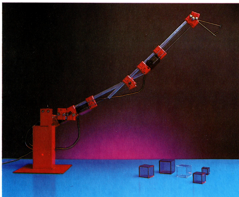
Name: Beasty Art: Roboterarm Programmierbar: Ja Software-Unterstützung: Ja Sensorische Rückmeldung? Position Vertrieb: Commotion Ltd., 241 Green Street, Enfield, Middlesex EN3 7SJ
