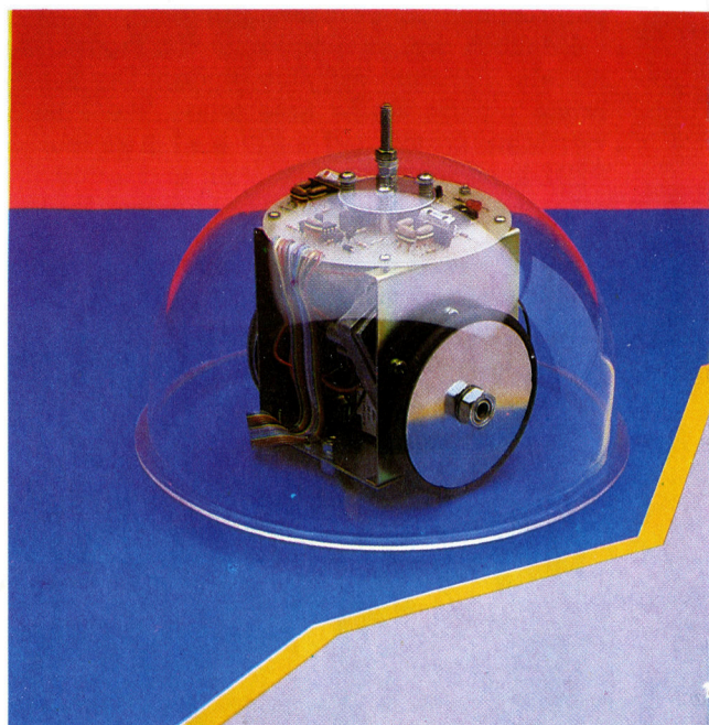
Name: Hebot II Typ: Bodenroboter Programmierbar: Ja Software-Unterstützung: Ja Sensorische Rückmeldung: Taster Hersteller: Powertran Cybernetics Ltd., West Portway Industrial Estate, Andover, Hampshire, SP 10 3NN
