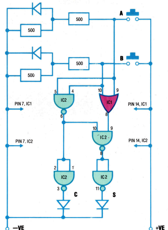
Elektrischer Schaltungsaufbau
